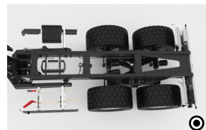
2 Vzpredni okvir iz profilnih cevi
