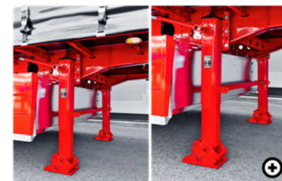
21 Podporne noge z izravnavo potiska Izravnavna potiska preprečuje upogibanje opornih nog pri spuščanju odložene polprikolice na zadnji strani.
