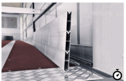
10 V-vtične letve z rebrom Te stranske vstavne letve imajo na vrhu in na dnu V-oblikovano izbočenje oziroma vdolbino. Tako jih je mogoče brez težav sestaviti v stransko steno.
